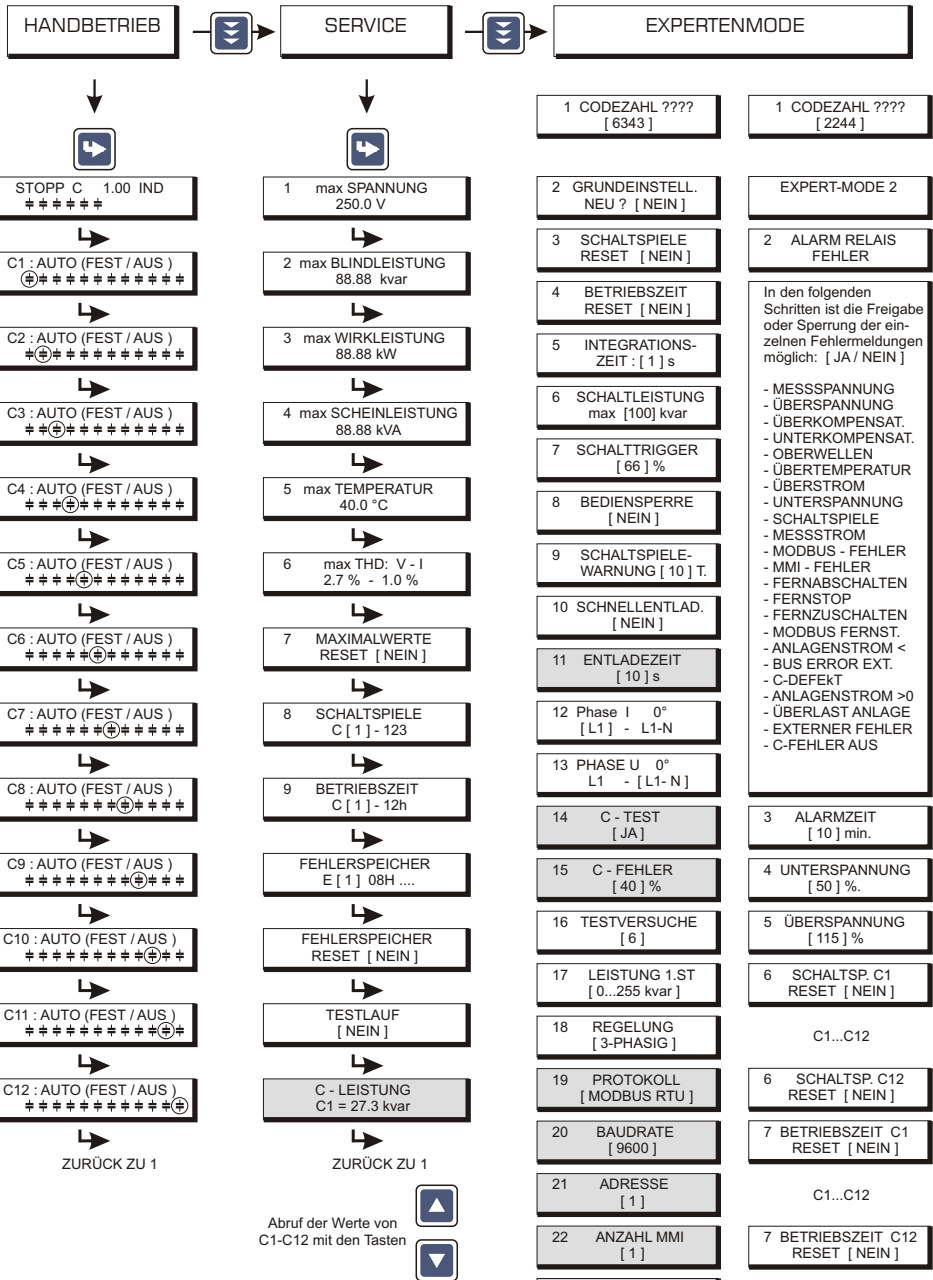
Bediendiagramm (Kurzreferenz) Blindleistungsregler BR 6000 (V5.1)
